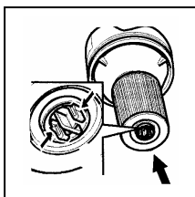
Ráncfilter
